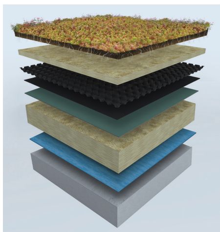
Teplá strecha na betónovom povrchu
