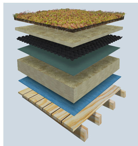
Teplá strecha na drevenej konštrukcii
