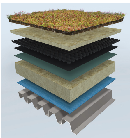
Teplá strecha na oceľovom povrchu
