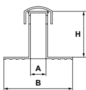
Jednoduchý
