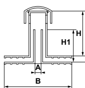
Dvojitý
